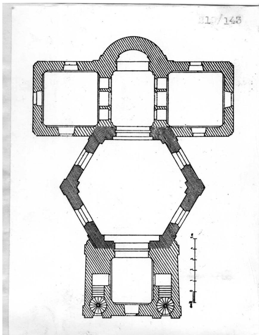
Snímek 219/143 Půdorys původní kaple z r. 1638 a přístavby v kostel z r. 1762 ↓
